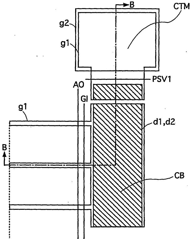
FIG.14B
