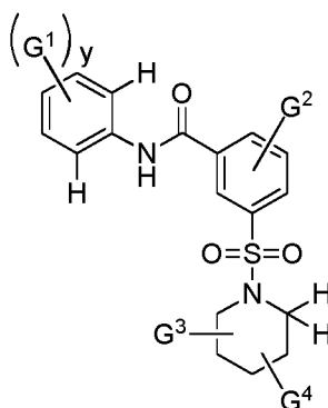
(IVb)
