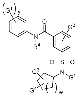
(VIa)
