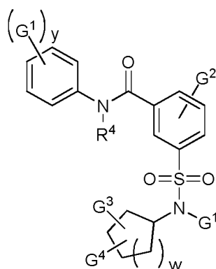
(VIa)
