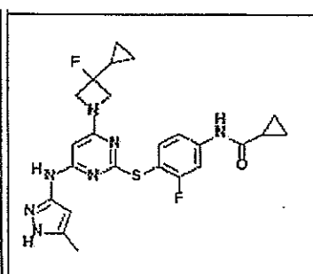
I-170
