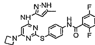
I-45
