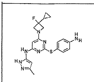
I-174
