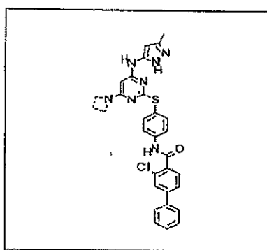
I-83
