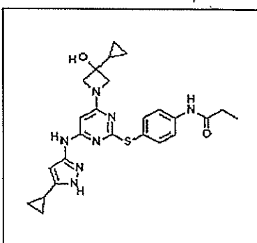
I-102
