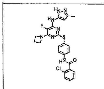
I-192
