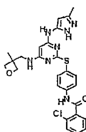
I-208
