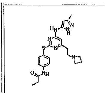
I-197
