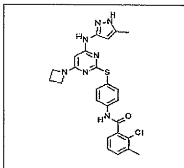
I-161
