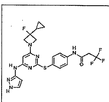
I-148
