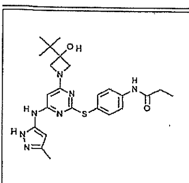
I-81
