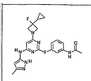
I-188
