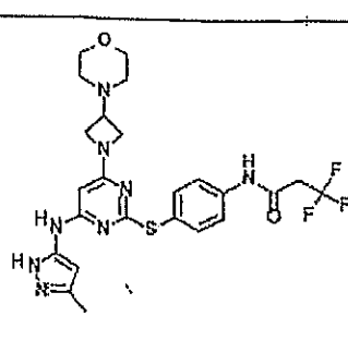
I-199
