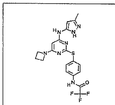
I-158
