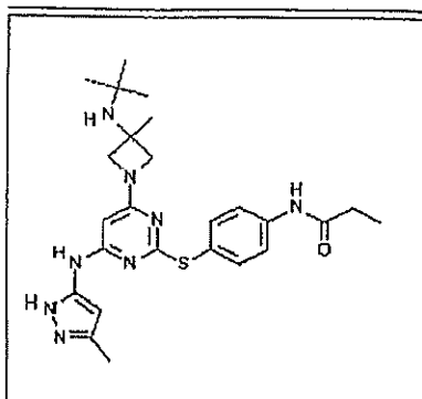
I-80
