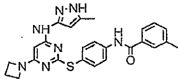
I-29
