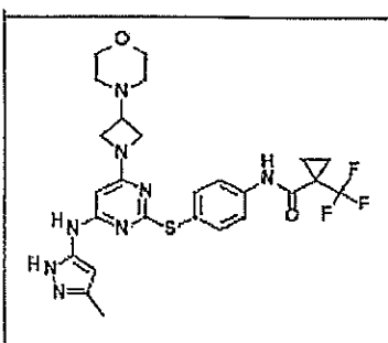
I-191
