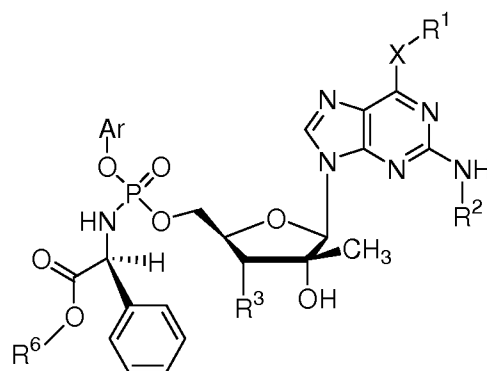
(XLIII)
