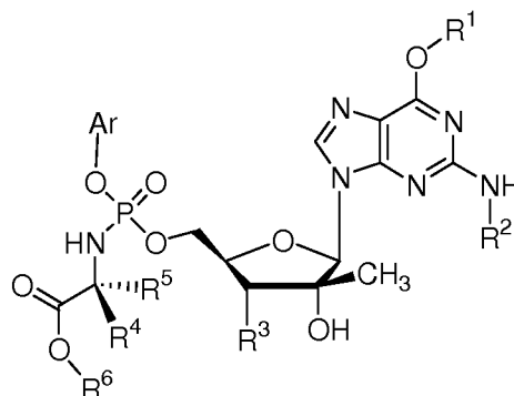
(XLIV)
