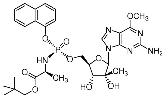
( R )-P
