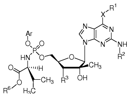
(XLII)
