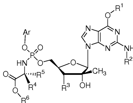
(XLIV)
