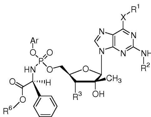
(XLIII)
