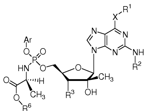
(XLI)
