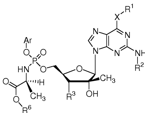
(XLI)
