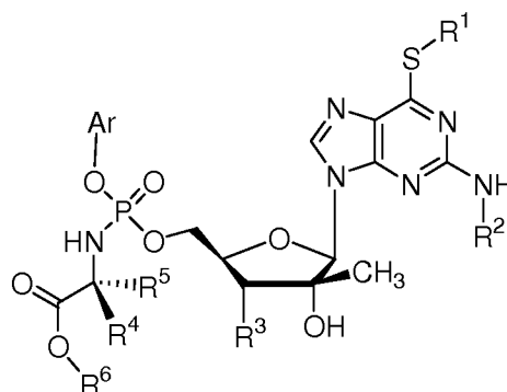
(XLVI)
