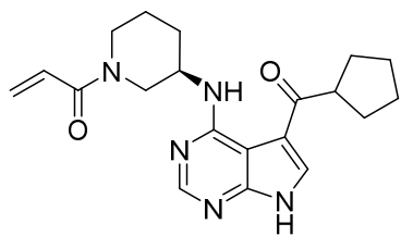
( R )-1-(3-((5-(cyclopentanecarbonyl)-7 H -pyrrolo[2,3- d ]pyrimidin-4-yl)amino)piperidin-1-yl)prop-2-en-1-one
