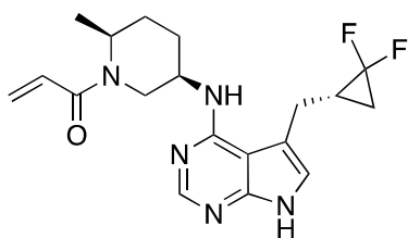
1-((2 S ,5 R )-5-((( S )-2,2-difluorocyclopropyl)methyl)-7 H -pyrrolo[2,3- d ]pyrimidin-4-yl)amino)-2-methylpiperidin-1-yl)prop-2-en-1-one ,
