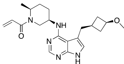
1-((2 S ,5 R )-5-(((1 S ,3 R )-3-methoxycyclobutyl)methyl)-7 H -pyrrolo[2,3- d ]pyrimidin-4-yl)amino)-2-methylpiperidin-1-yl)prop-2-en-1-one
