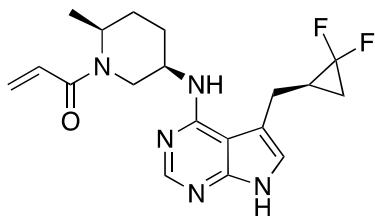
1-((2 S ,5 R )-5-((( R )-2,2-difluorocyclopropyl)methyl)-7 H -pyrrolo[2,3- d ]pyrimidin-4-yl)amino)-2-methylpiperidin-1-yl)prop-2-en-1-one ,
