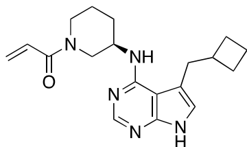
( R )-1-(3-((5-(cyclobutylmethyl)-7 H -pyrrolo[2,3- d ]pyrimidin-4-yl)amino)piperidin-1-yl)prop-2-en-1-one
