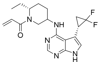
1-((2 R )-5-((5-(( S )-2,2-difluorocyclopropyl)-7 H -pyrrolo[2,3- d ]pyrimidin-4-yl)amino)-2-ethylpiperidin-1-yl)prop-2-en-1-one ,
