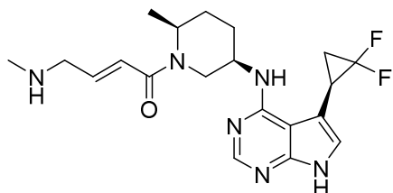
( E )-1-((2 S ,5 R )-5-((5-(( R )-2,2-difluorocyclopropyl)-7 H -pyrrolo[2,3- d ]pyrimidin-4-yl)amino)-2-methylpiperidin-1-yl)-4-(methylamino)but-2-en-1-one , and
