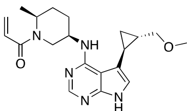
1-((2 S ,5 R )-5-(((1 S ,2 S )-2-(methoxymethyl)cyclopropyl)-7 H -pyrrolo[2,3- d ]pyrimidin-4-yl)amino)-2-methylpiperidin-1-yl)prop-2-en-1-one
