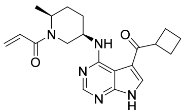
1-((2 S ,5 R )-5-((5-(cyclobutanecarbonyl)-7 H -pyrrolo[2,3- d ]pyrimidin-4-yl)amino)-2-methylpiperidin-1-yl)prop-2-en-1-one
