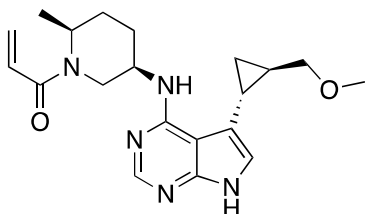
1-((2 S ,5 R )-5-(((1 R ,2 R )-2-(methoxymethyl)cyclopropyl)-7 H -pyrrolo[2,3- d ]pyrimidin-4-yl)amino)-2-methylpiperidin-1-yl)prop-2-en-1-one
