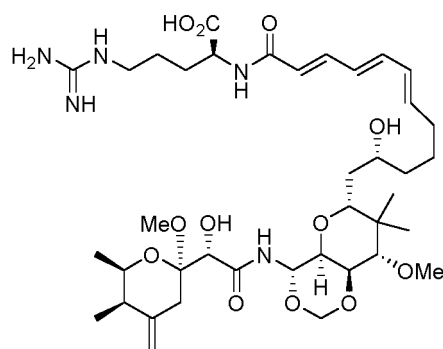
Onnamide A
