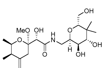
Mycalamide C
