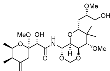
Mycalamide B
