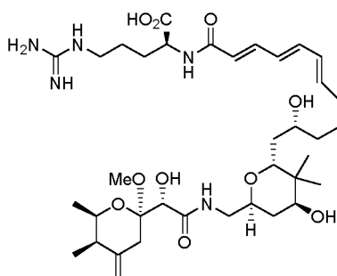
Onnamide E
