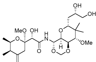
Mycalamide A
