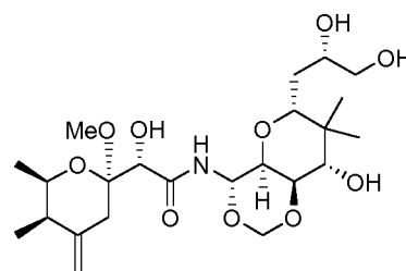
Mycalamide D
