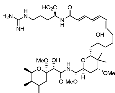
Onnamide D
