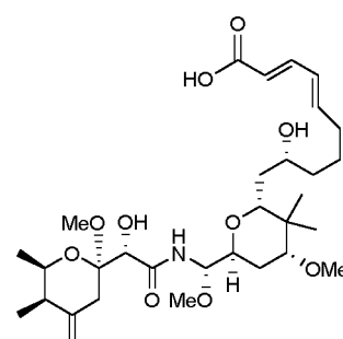
Onnamide F
