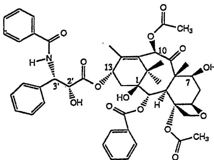
Paclitaxel
