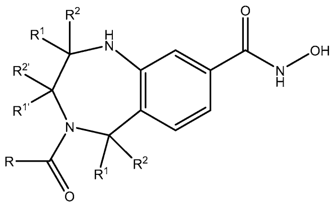
(IA-11).
