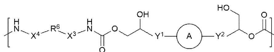
(VIIb)
