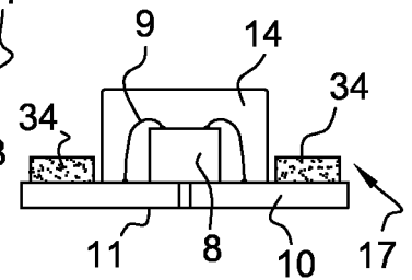
Fig. 5B Coupe B-B
