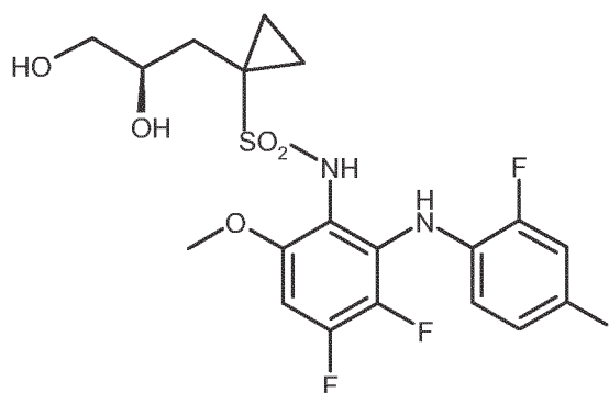
(R)-14 ;
