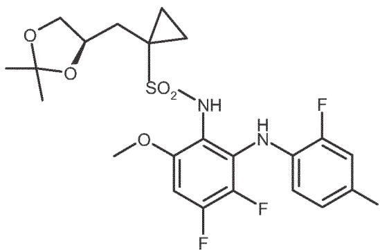
((R)-13)
