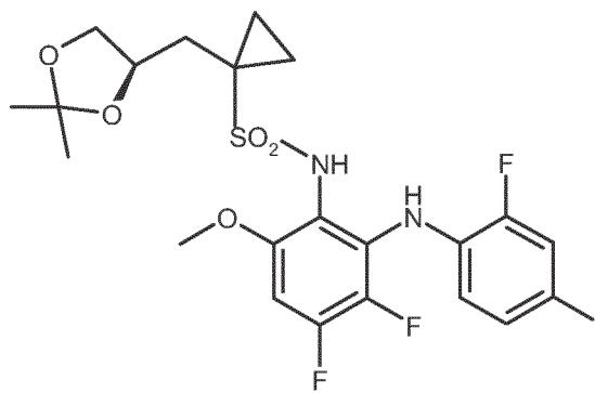
((R)-13)
