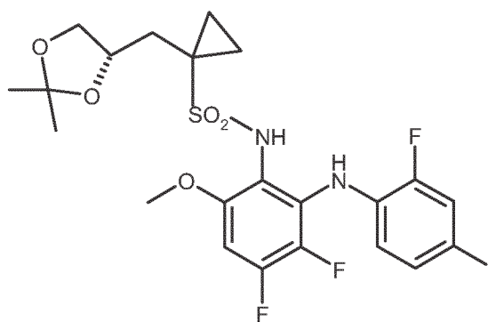
((S)-13)
