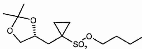
(R)-6 ;
