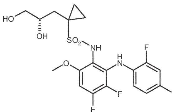
(S)-14 ;
