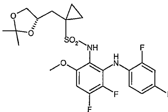
((S)-13)
