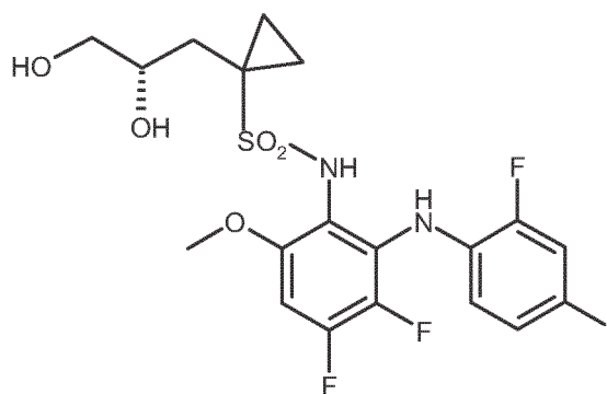
(S)-14 ;
