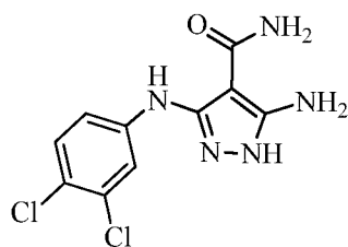
5-amino-3-((3,4-dichlorophenyl)amino)-1 H -pyrazole-4-carboxamide
