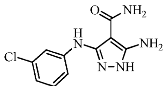
5-amino-3-((3-chlorophenyl)amino)-1 H -pyrazole-4-carboxamide
