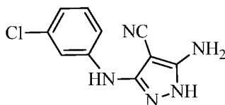
5-amino-3-((3-chlorophenyl)amino)-1 H -pyrazole-4-carbonitrile
