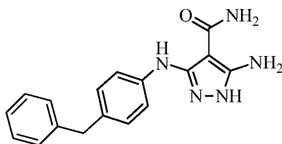
5-amino-3-((4-benzylphenyl)amino)-1H-pyrazole-4-carboxamide
