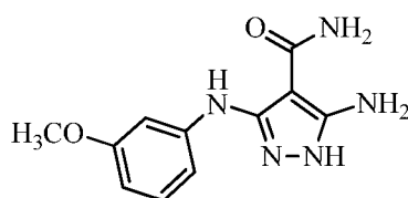
5-amino-3-((3-methoxyphenyl)amino)-1 H -pyrazole-4-carboxamide
