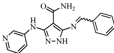
5-(benzylideneamino)-3-(pyridin-3-ylamino)-1 H -pyrazole-4-carboxamide
