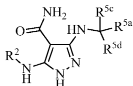
(XIV-c)
