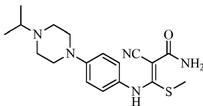
2-cyano-3-((4-(4-isopropylpiperazin-1-yl)phenyl)amino)-3-(methylthio)acrylamide
