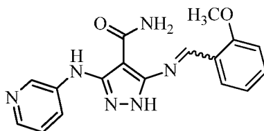
5-((2-methoxybenzylidene)amino)-3-(pyridin-3-ylamino)-1 H -pyrazole-4-carboxamide
