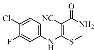
3-((4-chloro-3-fluorophenyl)amino)-2-cyano-3-(methylthio)acrylamide
