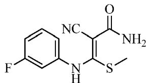
2-cyano-3-((3-fluorophenyl)amino)-3-(methylthio)acrylamide
