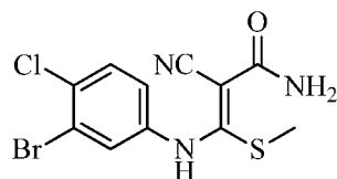
3-((3-bromo-4-chlorophenyl)amino)-2-cyano-3-(methylthio)acrylamide
