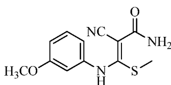
2-cyano-3-((3-methoxyphenyl)amino)-3-(methylthio)acrylamide
