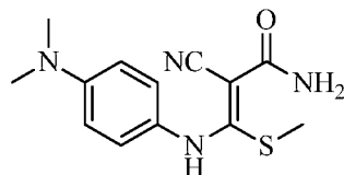
2-cyano-3-((4-(dimethylamino)phenyl)amino)-3-(methylthio)acrylamide
