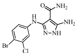
5-amino-3-((4-bromo-3-chlorophenyl)amino)-1H-pyrazole-4-carboxamide
