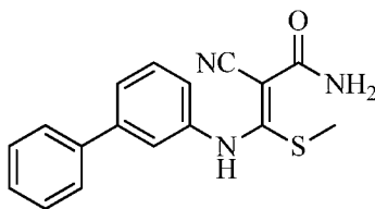
3-([1,1'-biphenyl]-3-ylamino)-2-cyano-3-(methylthio)acrylamide
