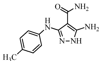
5-amino-3-( p -tolylamino)-1 H -pyrazole-4-carboxamide
