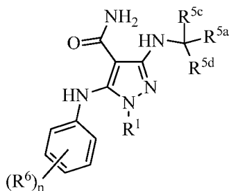
(XVII-b)
