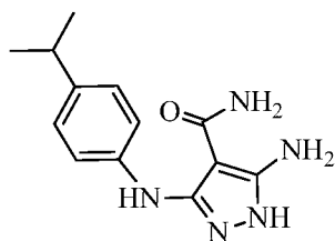
5-amino-3-((4-isopropylphenyl)amino)-1 H -pyrazole-4-carboxamide
