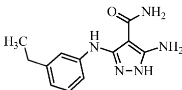
5-amino-3-((3-ethylphenyl)amino)-1 H -pyrazole-4-carboxamide
