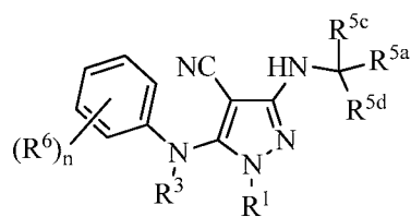
(XVI)
