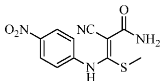
2-cyano-3-(methylthio)-3-((4-nitrophenyl)amino)acrylamide
