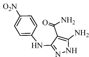
5-amino-3-((4-nitrophenyl)amino)-1 H -pyrazole-4-carboxamide
