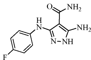
5-amino-3-((4-fluorophenyl)amino)-1 H -pyrazole-4-carboxamide
