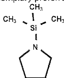
Trimethylsilylpyrrolidine
