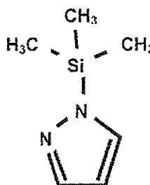
Trimethylsilylpyrazole
