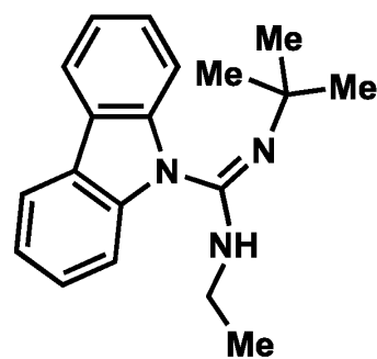
Ligand 11
