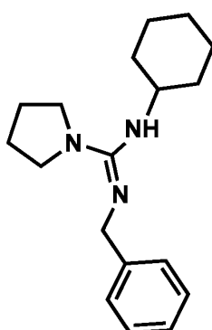
Ligand 2
