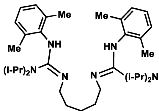
Ligand 17
