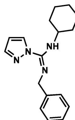
Ligand 6
