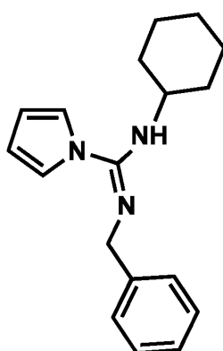
Ligand 5
