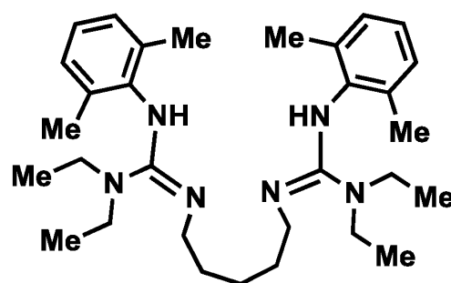
Ligand 16
