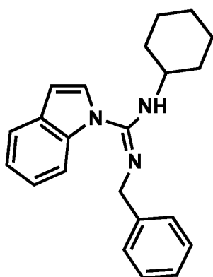
Ligand 4
