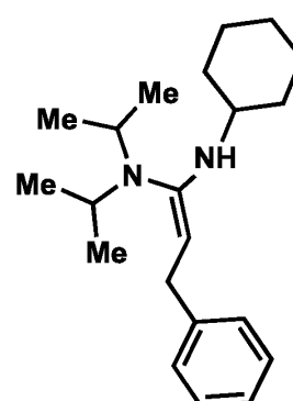
Ligand 3
