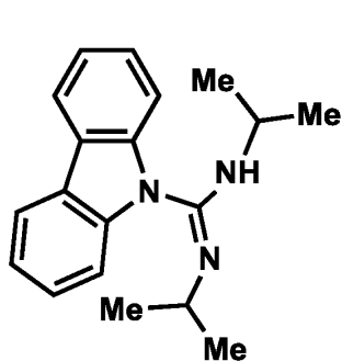
Ligand 8
