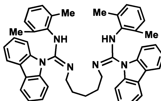
Ligand 14
