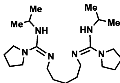
Ligand 12
