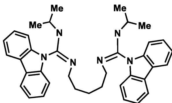
Ligand 15
