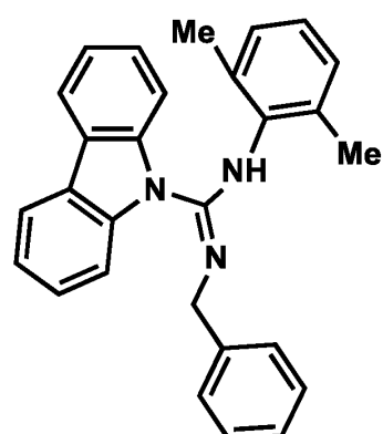
Ligand 9
