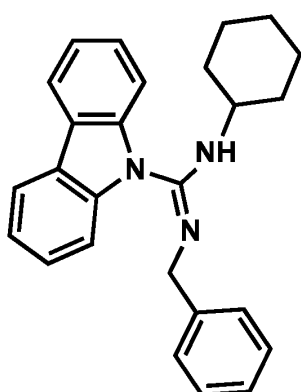
Ligand 7
