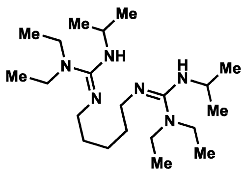
Ligand 13
