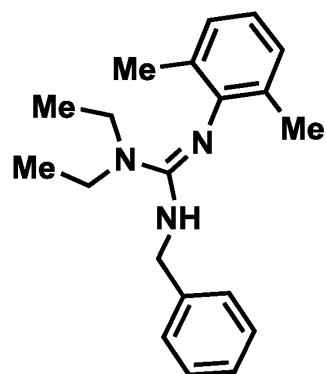
Ligand 10
