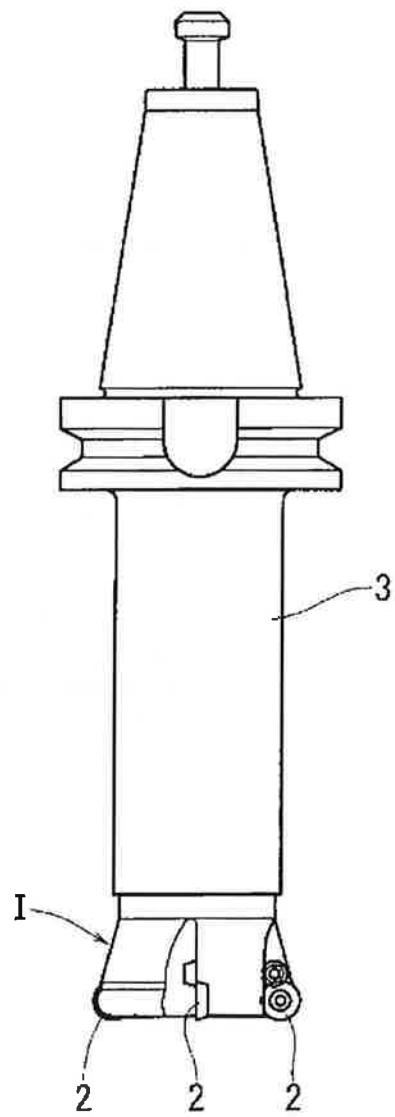
FIG.11B
