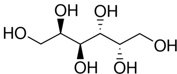
Dulcitol,
