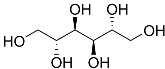
Mannitol,
