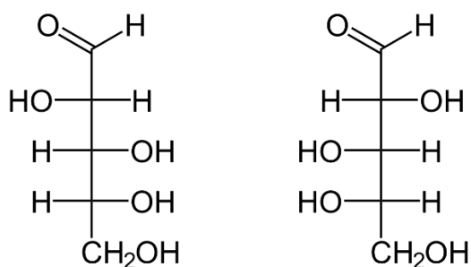
D-Arabinose
