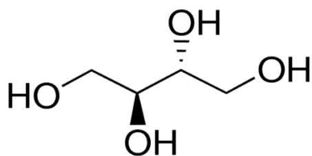
Meso-erythritol,
