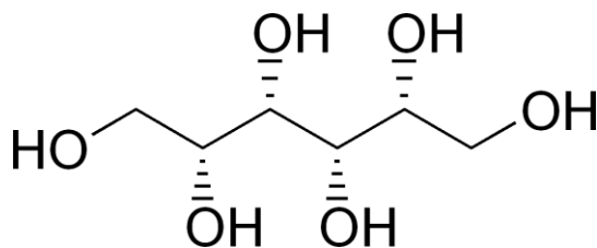
Iditol,
