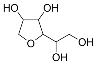
Sorbitan,
