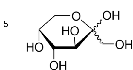
10 D- (-)-Fructose,
