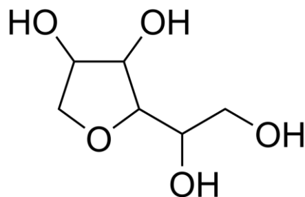
Sorbitan,
