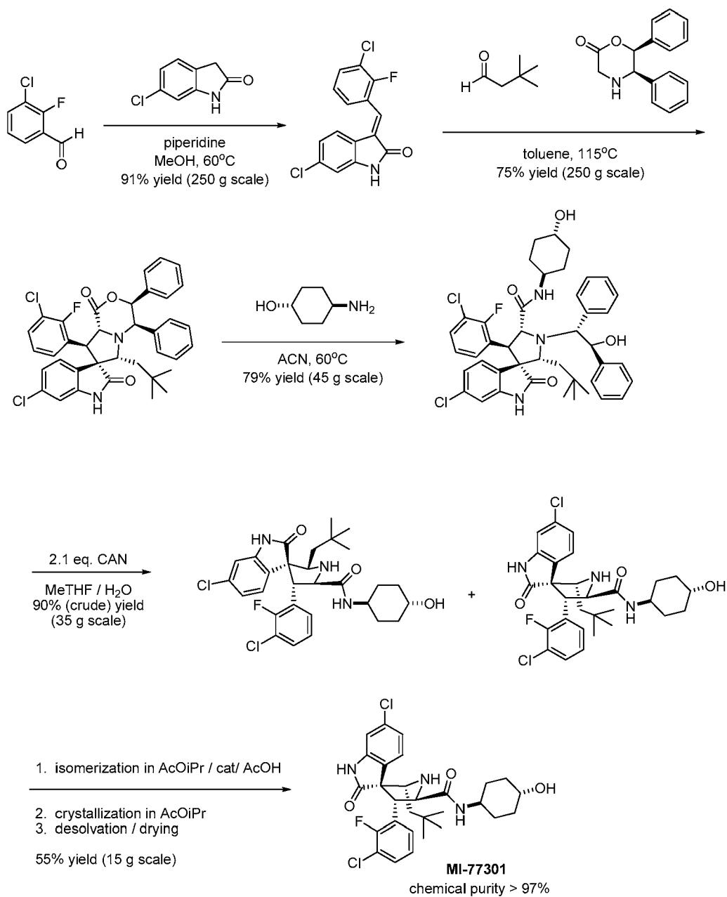
Scheme 9A
