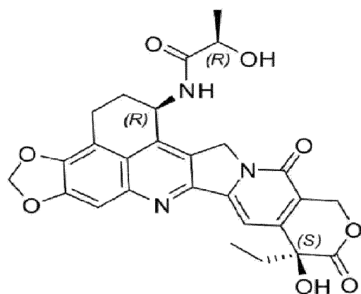
[화학식 8]
