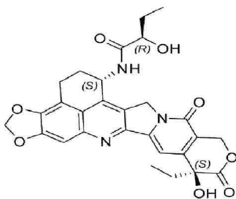
[화학식 10]
