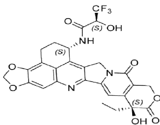
[화학식 9]
