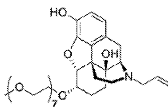
naloxegol
