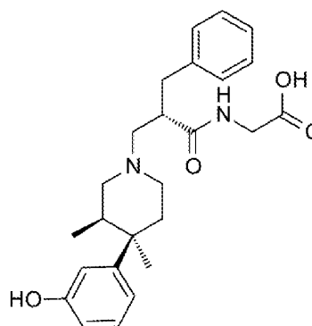
alvimopan
