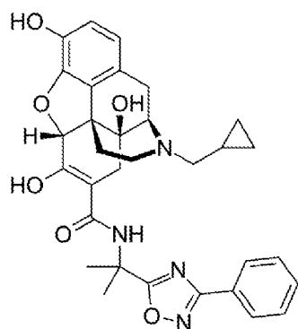
naldemedine
