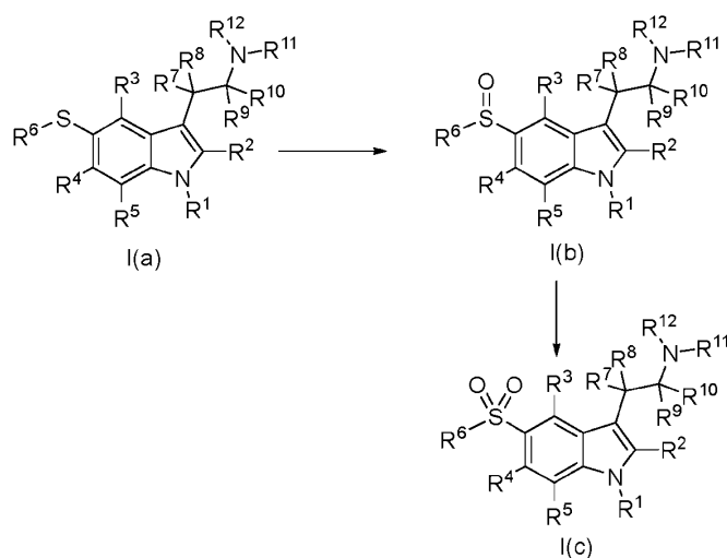
Scheme VI
