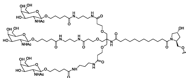
GalNAc L96
