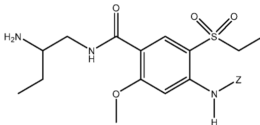
Formula IC
