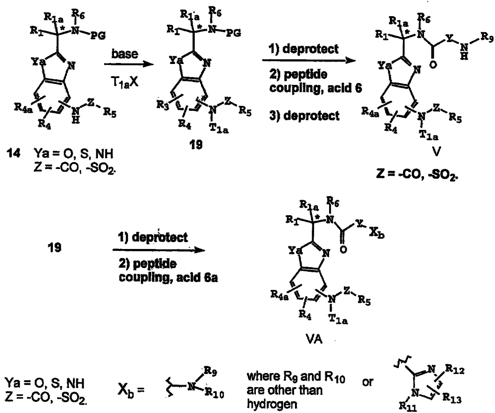
Scheme 1e
