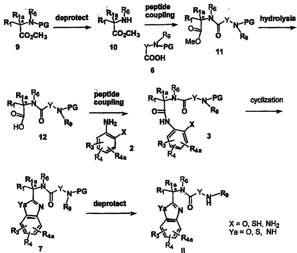
Scheme 1a
