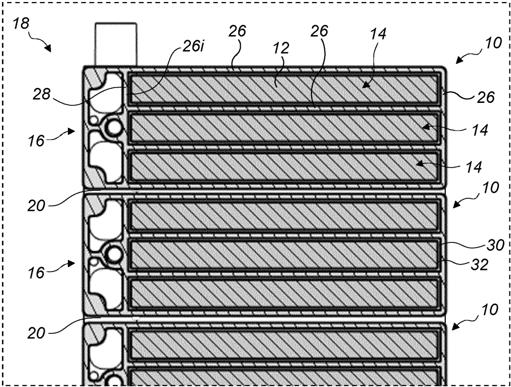
FIG. 3 A-A
