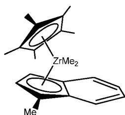
(CpMe5)(1-MeInd)ZrMe2
