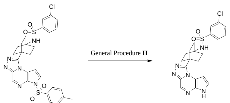
Example #H.1.1
