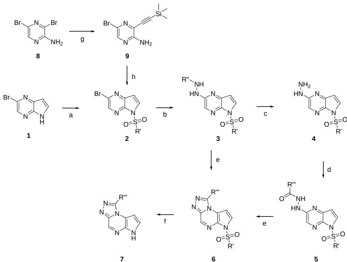
Scheme I:
