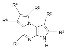
Formula (Id) ,
