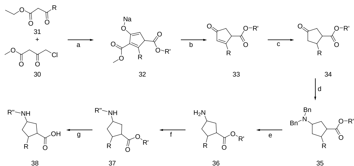
Scheme VI
