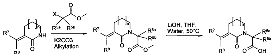
Scheme 8-1:
