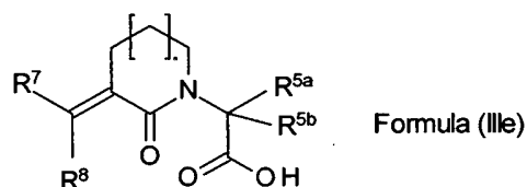
Scheme 8-1:
