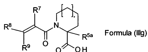
10 Scheme 10-1:
