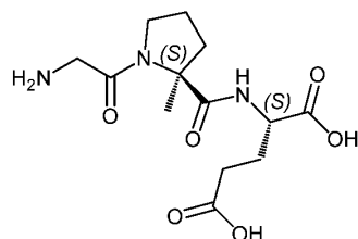
(Ia) (trofinetide),
