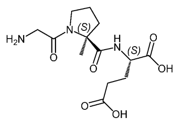
(Ia) (trofinetide),
