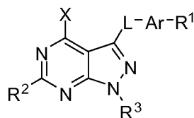
Formula (IA);
