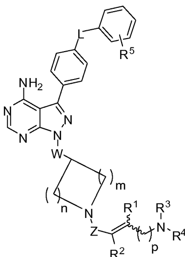
Formula (VIA);
