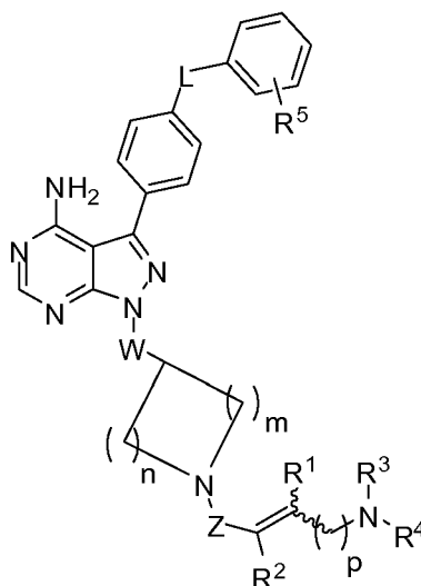
Formula (VI);
