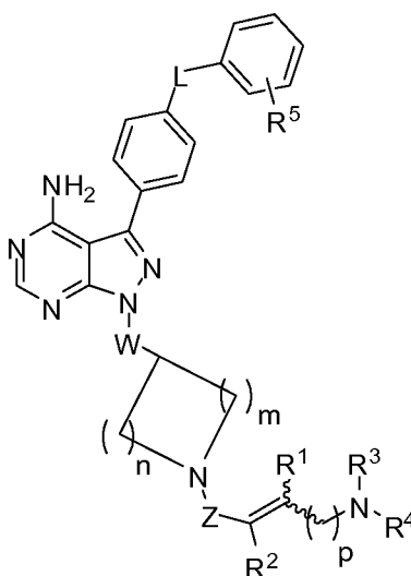
Formula (VIA);
