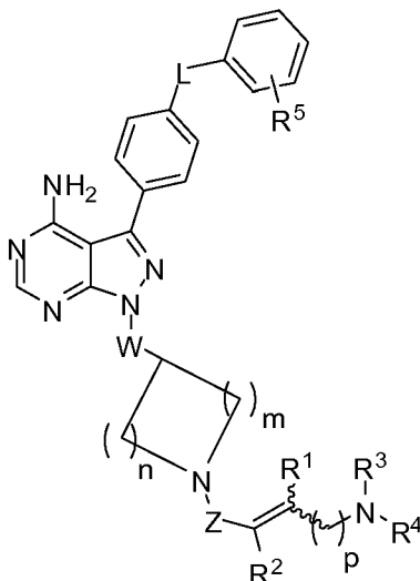
Formula (VI);
