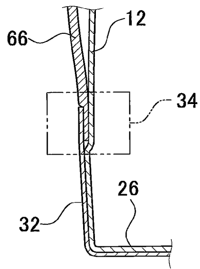
Ⅱ-Ⅱ 端断面
