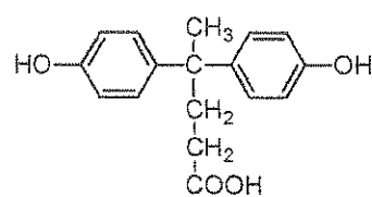
BisP-LV
