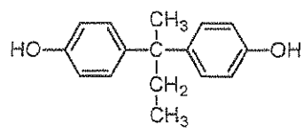
BisP-B
