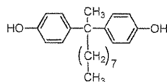
BisP-DE
