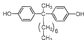
BisP-NO
