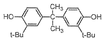
BisOTBP-A
