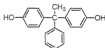
BisP-AP
