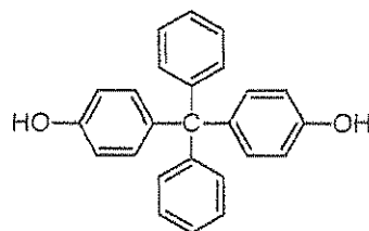
BisP-DP
