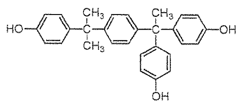
TrisP-PA
