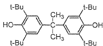
Bis26B-A
