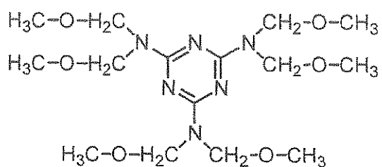
NIKALAC MW-30HM
