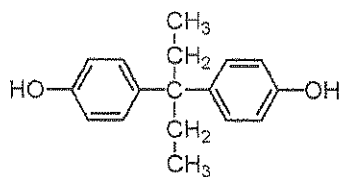
BisP-DEK
