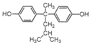
BisP-MBK
