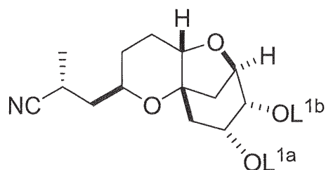
(Ib)
