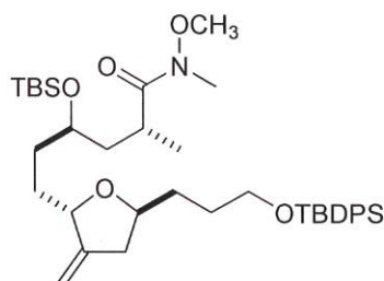
Compound AV
