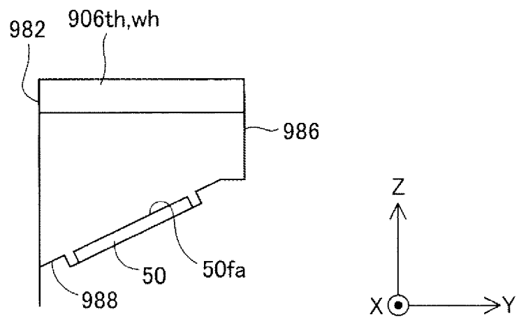
45-45断面図
