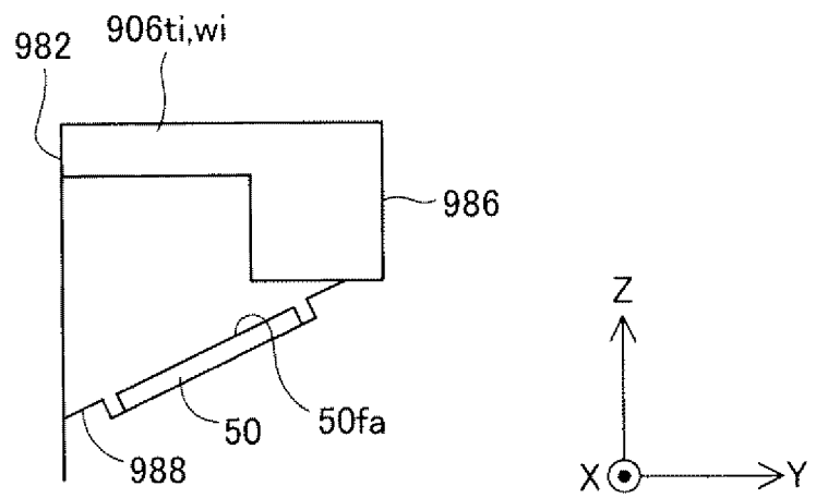
46-46断面図
