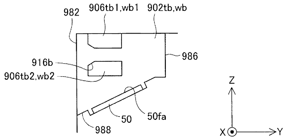
39-39断面図
