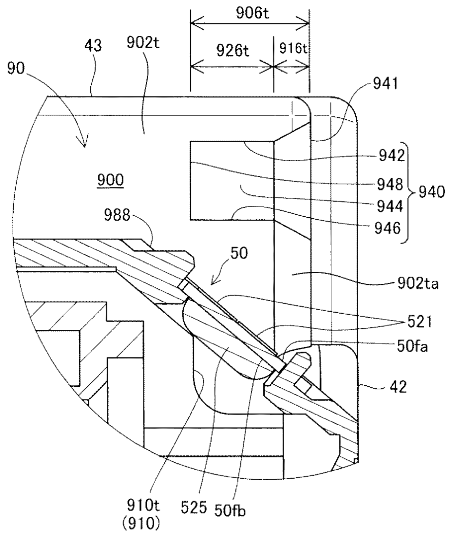
28b-28b断面図
