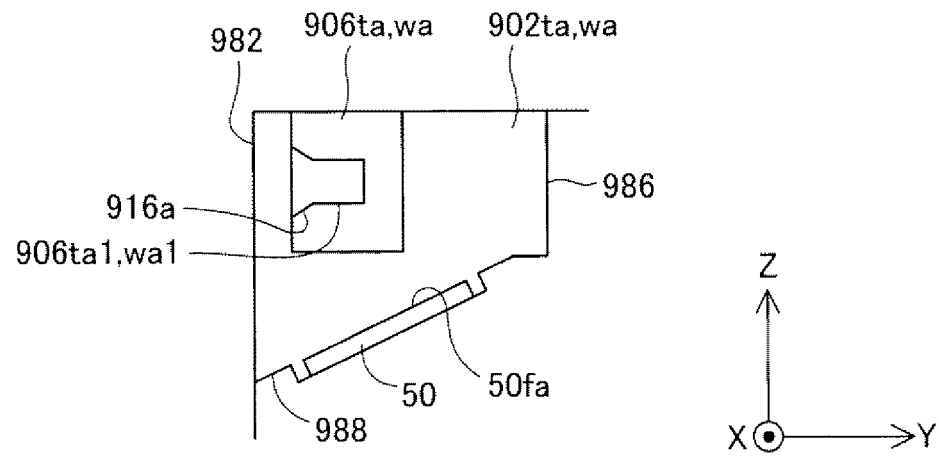
38-38断面図
