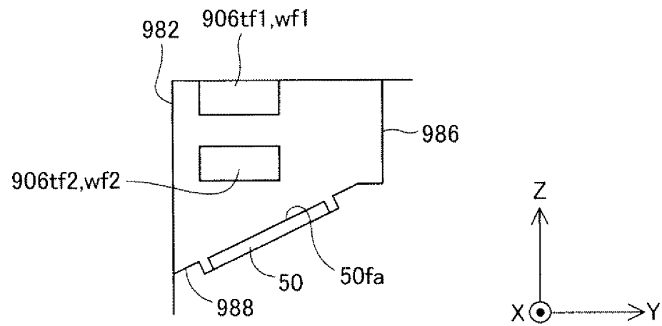
43-43断面図
