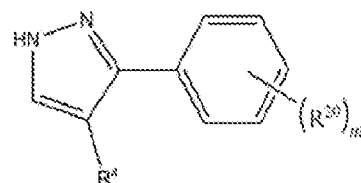
Formula (IXar);
