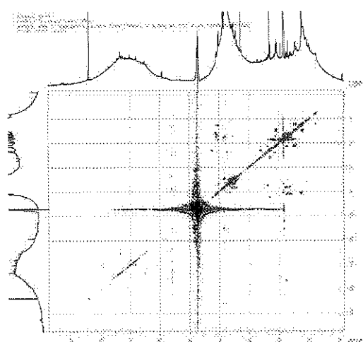
^1\text{H} , ^1\text{H} -COSY
