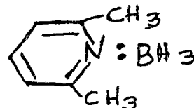
2,6-lutidine borane
