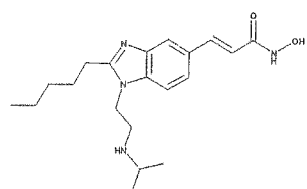
N-Hydroxy-3-[1-(2-isopropylamino-ethyl)-2-pentyl-1H-benzoimidazol-5-yl]-acrylamide
