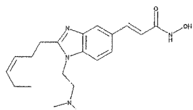
3-[1-(2-Dimethylamino-ethyl)-2-hex-3-enyl-1H-benzoimidazol-5-yl]-N-hydroxy-acrylamide
