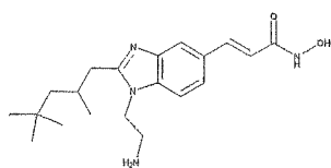
3-[1-(2-Amino-ethyl)-2-(2,4,4-trimethyl-pentyl)-1H-benzoimidazol-5-yl]-N-hydroxy-acrylamide
