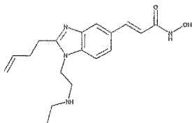
3-[2-But-3-enyl-1-(2-ethylamino-ethyl)-1H-benzoimidazol-5-yl]-N-hydroxy-acrylamide
