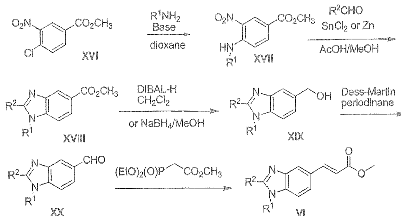
Scheme VI
