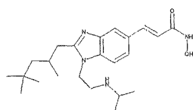
N-Hydroxy-3-[1-(2-isopropylamino-ethyl)-2-(2,4,4-trimethyl-pentyl)-1H-benzoimidazol-5-yl]-acrylamide
