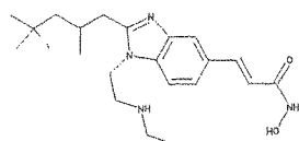
3-[1-(2-Ethylamino-ethyl)-2-(2,4,4-trimethyl-pentyl)-1H-benzoimidazol-5-yl]-N-hydroxy-acrylamide
