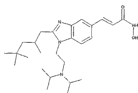
3-[1-(2-Diisopropylamino-ethyl)-2-(2,4,4-trimethyl-pentyl)-1H-benzoimidazol-5-yl]-N-hydroxy-acrylamide
