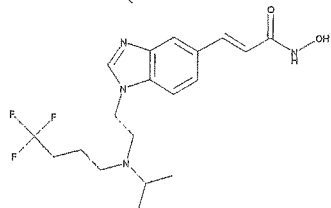
(E)-N-hydroxy-3-(1-(2-(isopropyl(4,4,4- trifluorobutyl)amino)ethyl)-1H-benzimidazol- 5-yl)acrylamide
