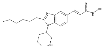
3-(2-Hexyl-1-piperidin-3-yl-1H-benzoimidazol-5-yl)-N-hydroxy-acrylamide
