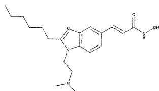
3-[1-(2-Dimethylamino-ethyl)-2-hexyl-1H-benzoimidazol-5-yl]-N-hydroxy-acrylamide
