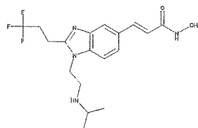
N-Hydroxy-3-[1-(2-isopropylamino-ethyl)-2-(3,3,3-trifluoro-propyl)-1H-benzoimidazol-5-yl]-acrylamide
