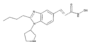
3-(2-Butyl-1-pyrrolidin-3-yl)-1H-benzoimidazol-5-yl)-N-hydroxy-acrylamide
