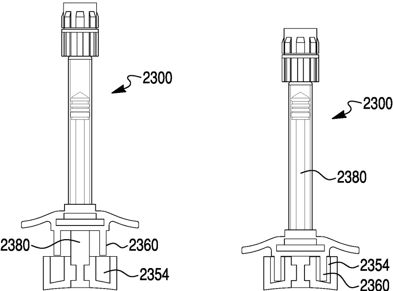
FIG. 27G FIG. 27H
