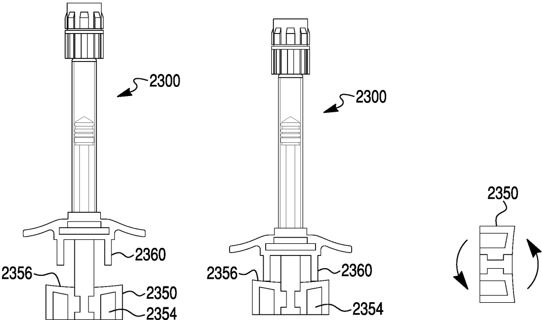
FIG. 27D FIG. 27E FIG. 27F
