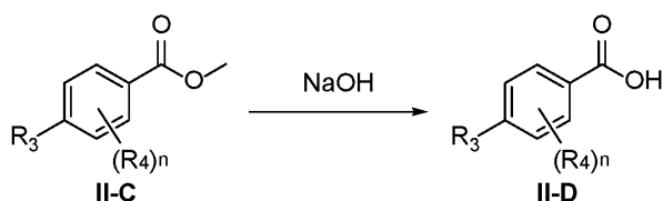
SCHEME II-2
