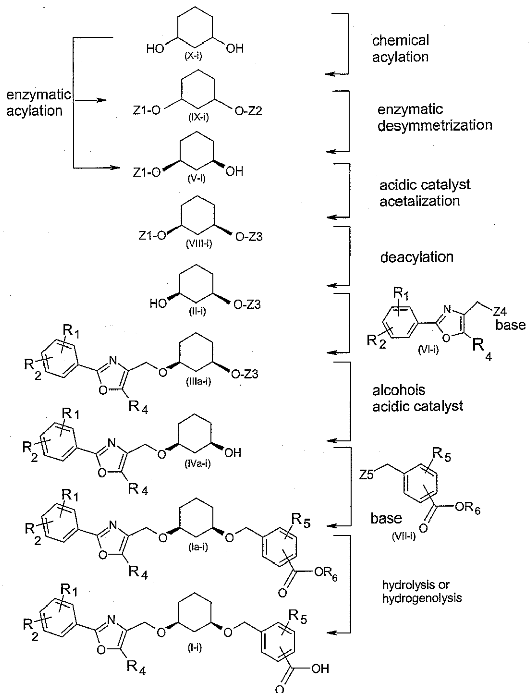
Scheme II:
