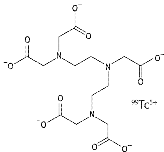
^{99m}\text{Tc-DTPA}
