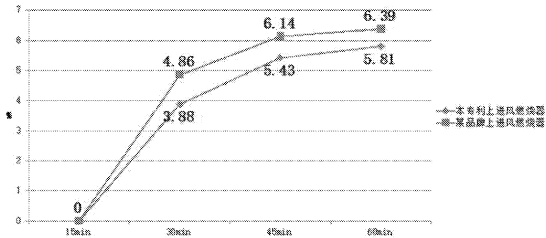
本专利与某品牌上进风燃烧器(12T)燃烧15-60min 热负荷下降率对比图
