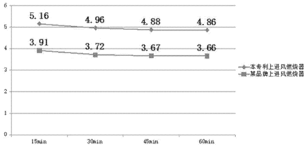
本专利与某品牌上进风燃烧器(12T)燃烧15-60min 热负荷变化对比图
