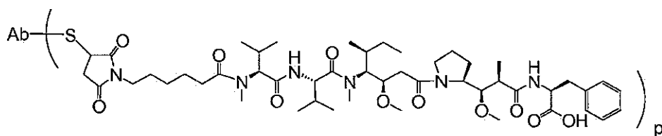
Ab-MC-MMAF
