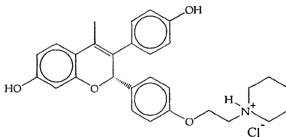
Acolbifene (EM-652.HCl; EM-1538)
