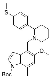
中间体3:
