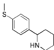
中间体2:
