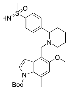
中间体4:
