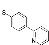
中间体1:
