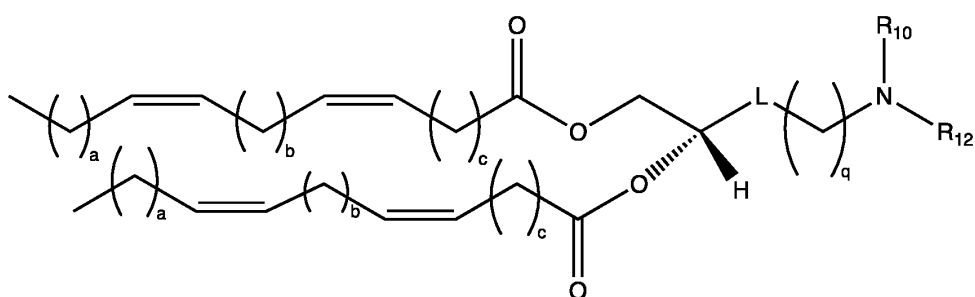
Formula I-A
