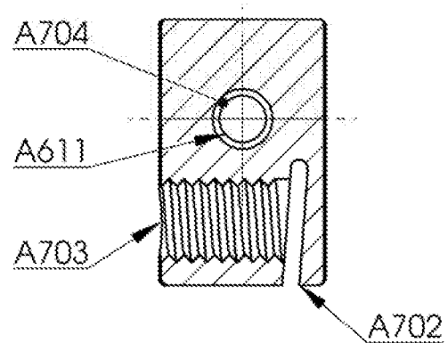
FIG. A7f SECTION B-B
