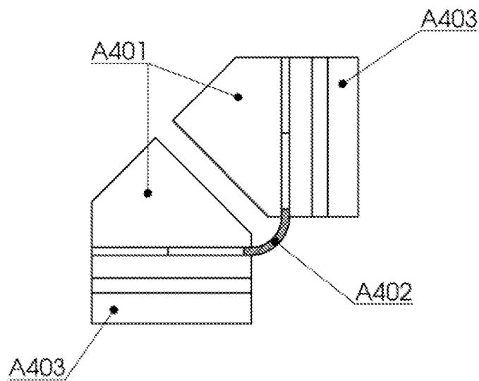
FIG. A4d SECTION A-A
