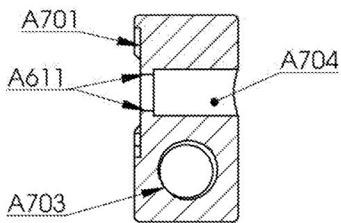
FIG. A7e SECTION A-A
