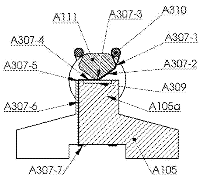
FIG. A3h SECTION B-B
