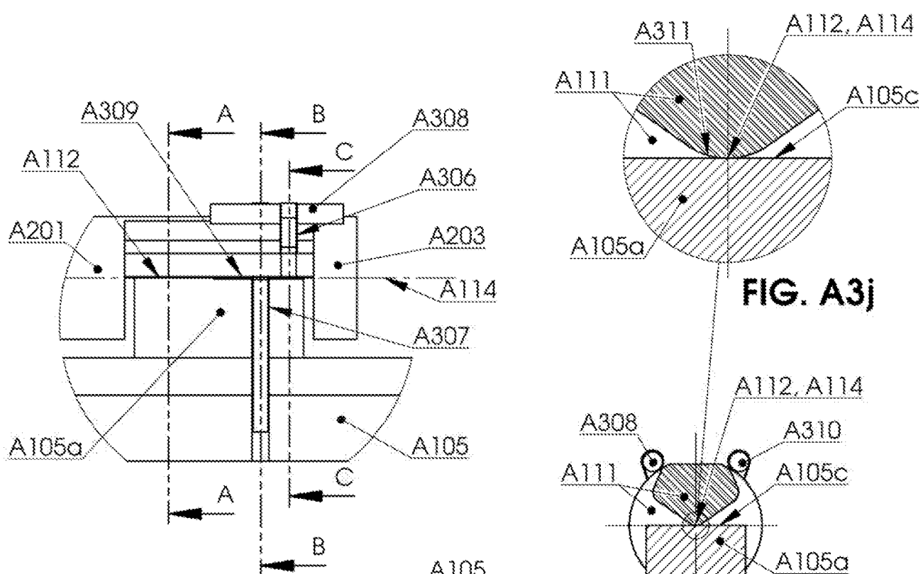
FIG. A3f DETAIL A
