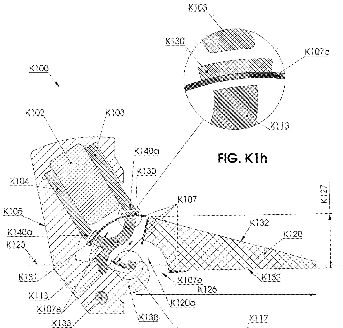
FIG. K1g SECTION A-A
