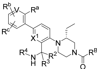
Formula (IXa).
