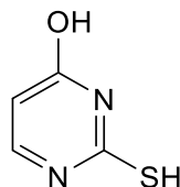
2-mercaptopyrimidin-4-ol (VIVm)
