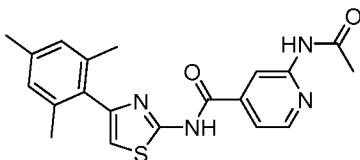
2-Acetamido-N-(4-mesitylthiazol-2-yl)isonicotinamide
